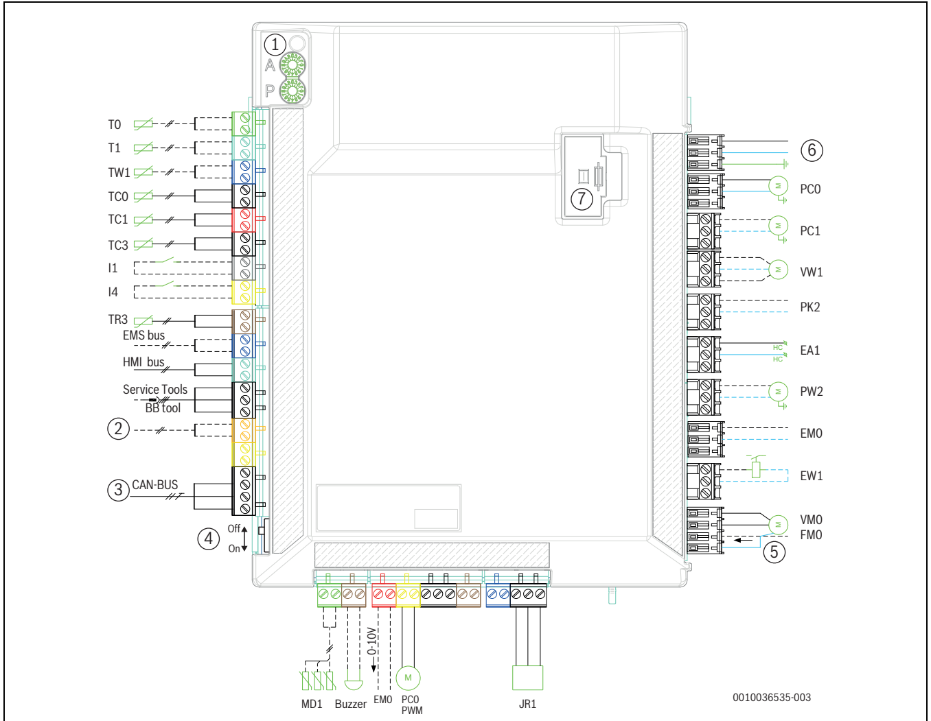
37. ábra A beltéri egység telepítői modulja
