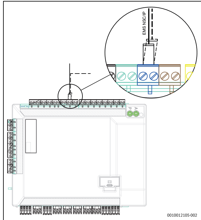
20. ábra EMS-csatlakoztatás a szerelőmodulra
