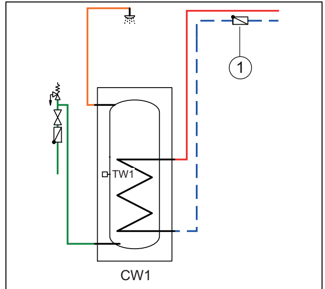
21. ábra Melegvítároló
