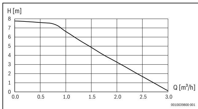
29. ábra Primer keringetőszivattyú (PCO) teljesítménygörbéje
