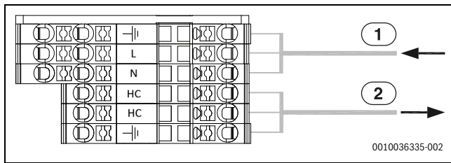
16. ábra Elektromos csatlakozások
