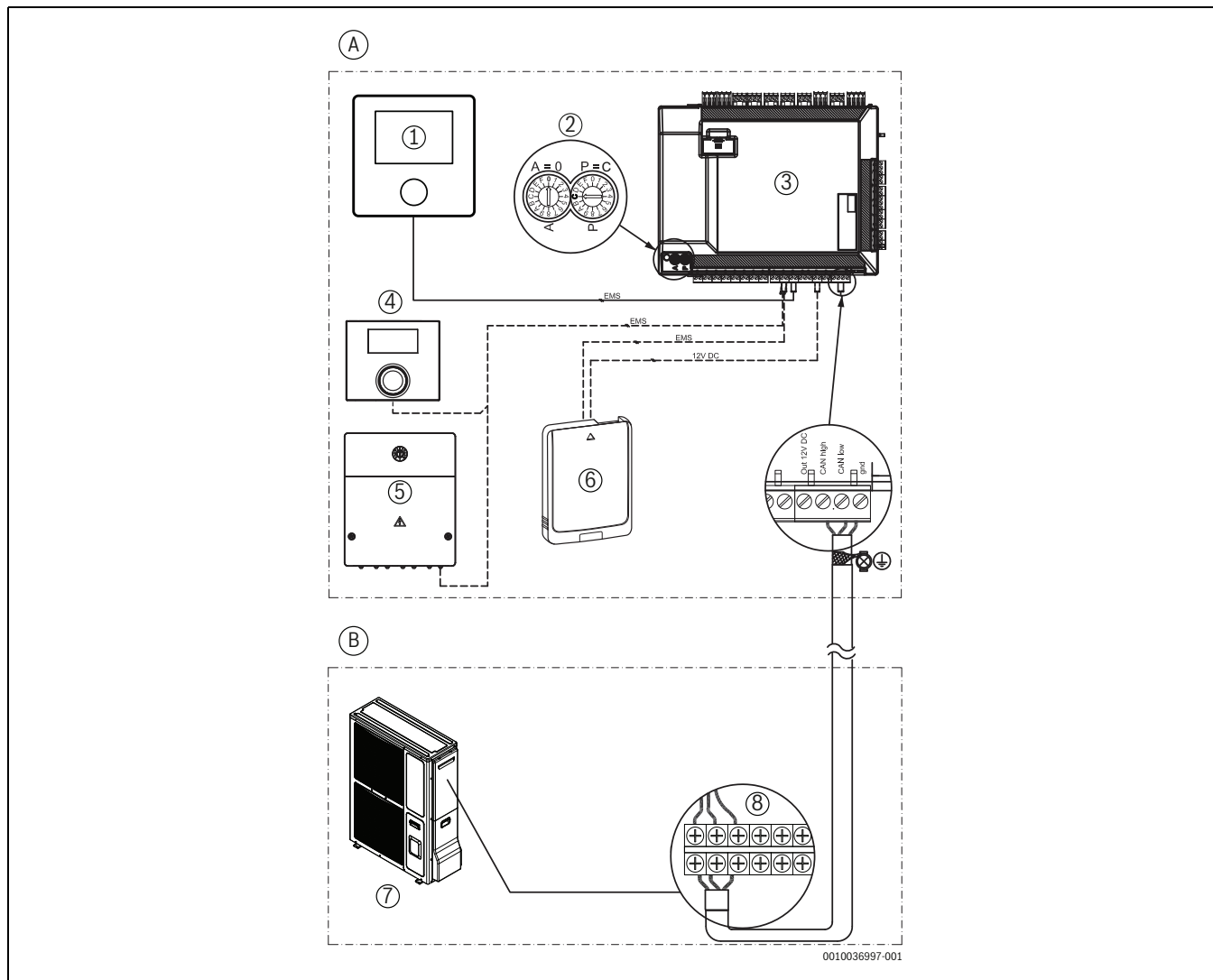
38. ábra CAN és EMS csatlakozások
